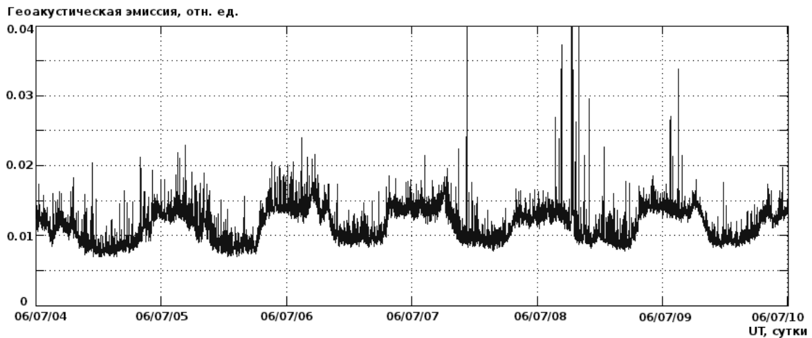
Рис. 1. Исходный геоакустический сигнал в диапазоне частот от 2000 до 6500 Гц
