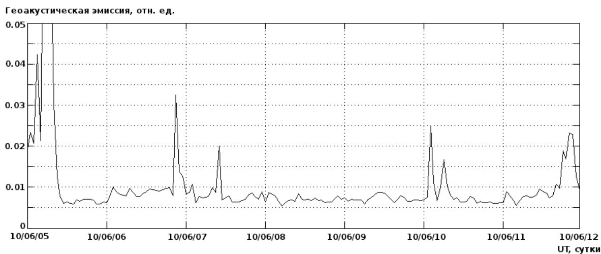
Рис. 3. Участок данных, на котором суточный ход ГАЭ не наблюдается
