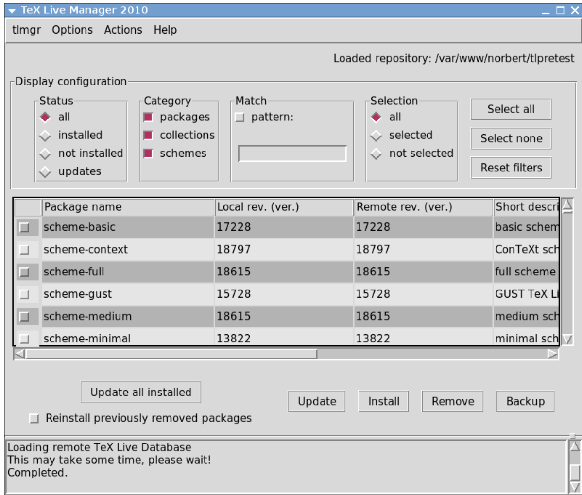
Рис. 8: tlmgr в графическом режиме. Список пакетов/коллекций/схем виден только после нажатия на клавишу «Load»
