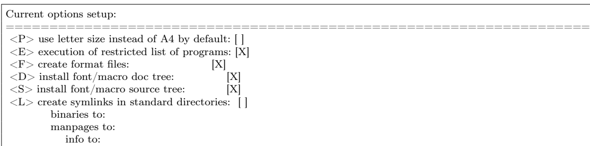
Рис. 7: Меню опций (Unix)
