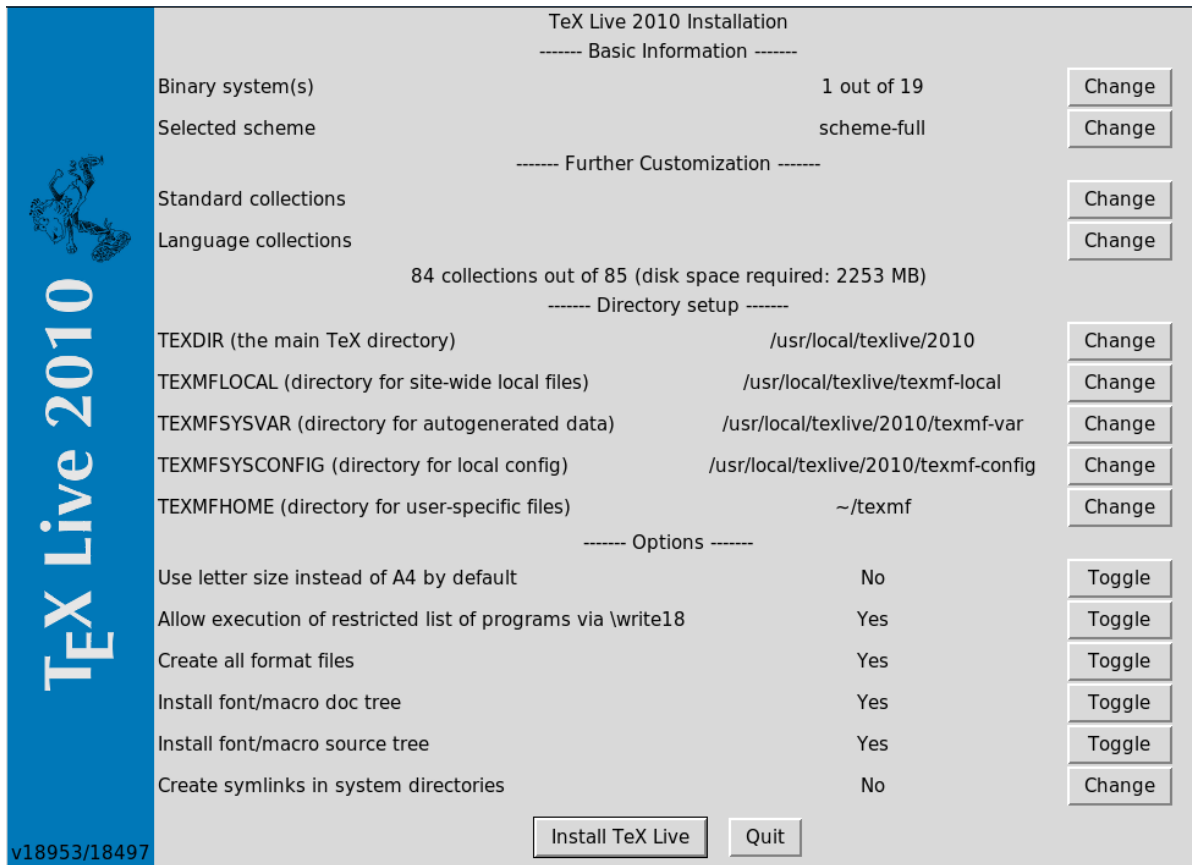
Рис. 2: Главное меню программы установки в экспертном графическом режиме (GNU/Linux)
